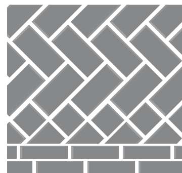
▶ Fischgrätverband mit Bischofsmützen – zur Angrenzung an einen linearen Rahmen
