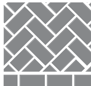
▶ Fischgrätverband mit Anschluss – Teilstücke mit geschnittenen Steinen zur Anbindung an den Rahmen der Fläche
