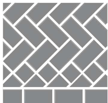
▶ Fischgrätverband mit Anschluss – Teilstücke mit halben Steinen zur Anbindung an den Rahmen der Fläche
