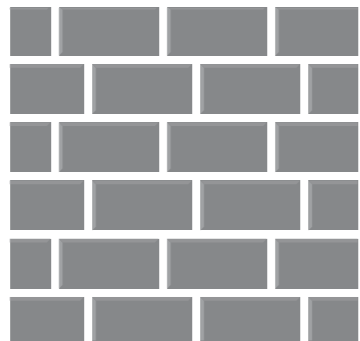
▶ Läuferverband – Viertel Stein versetzt: geringere Verbundwirkung, die das Gesamtbild auflockert
