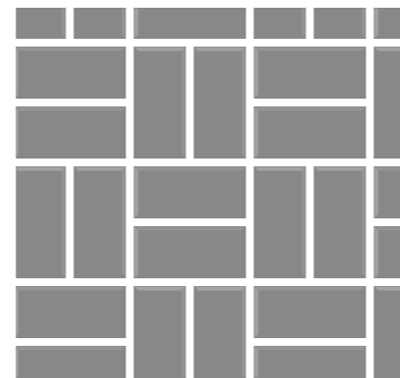
▶ Blockverband – Für eine geordnete und doch in sich selbst unterschiedliche Verlegung von Pflastersteinen
