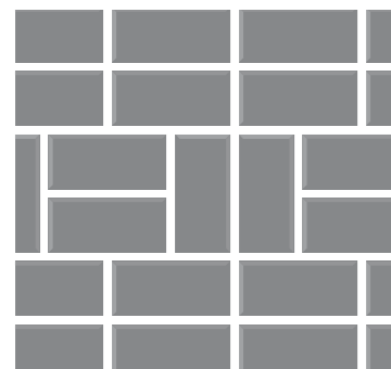
▶ Blockverband – aufgelockerte Variante der starren Blockverbandverlegung
